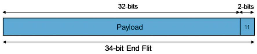
Fig. 4.37 END flit format
